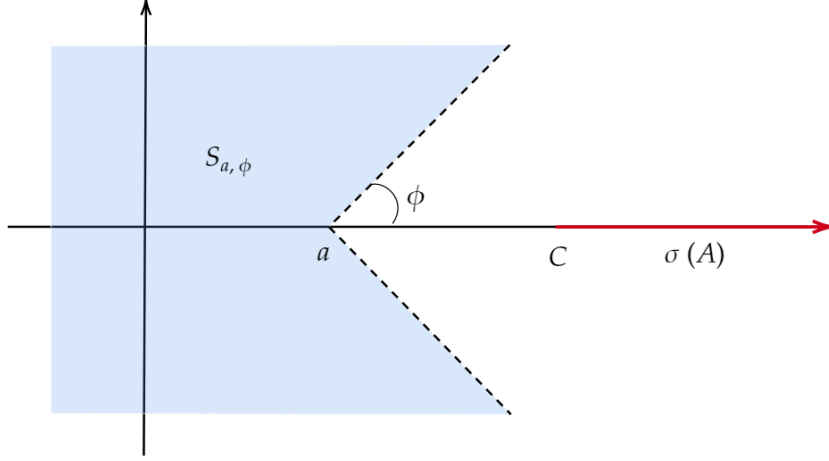
Figura 1.5: Representação do setor S_{a,\phi} para a = C/2 e \phi = \pi/4 .
