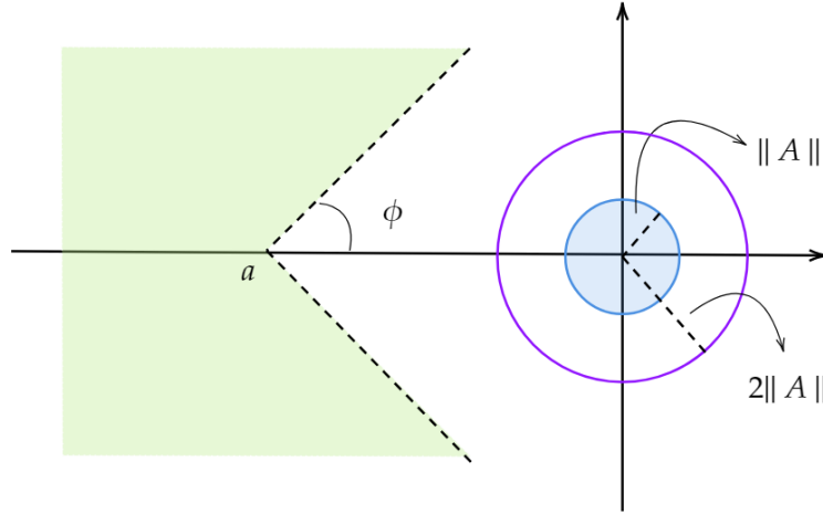
Figura 1.4: Representação do setor S_{a,\phi} para a \leq -3\|A\| e \phi = \frac{\pi}{4} .
