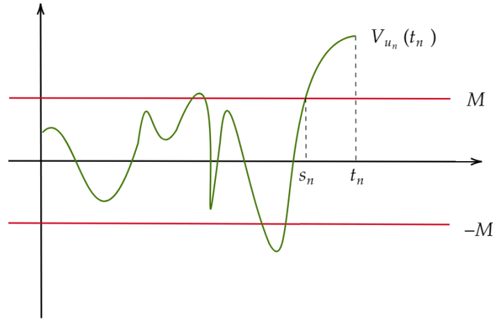
Figura 3.1: Boa definição de s_n .
