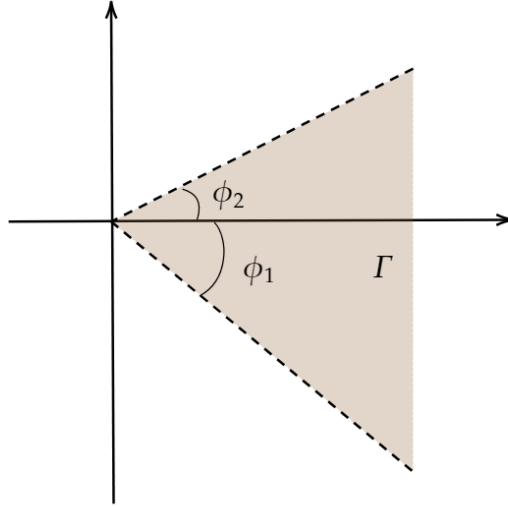
Figura 1.1: Representação geométrica do setor \Gamma .
