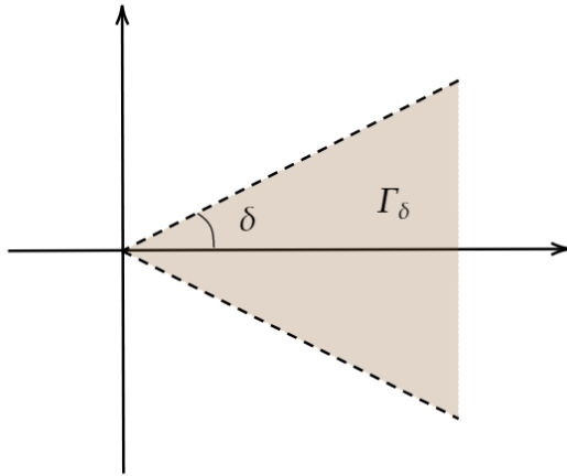
Figura 1.2: Representação geométrica do setor \Gamma_\delta .
