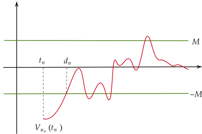
Figura 3.2: Boa definição de d_n .
