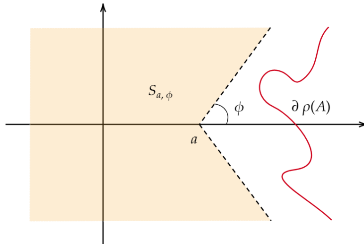
Figura 1.3: Representação do setor S_{a,\phi} .
