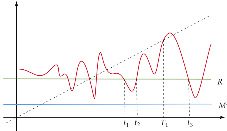
Figura 3.3: Definição das seqüências (t_n) e (T_n) .
