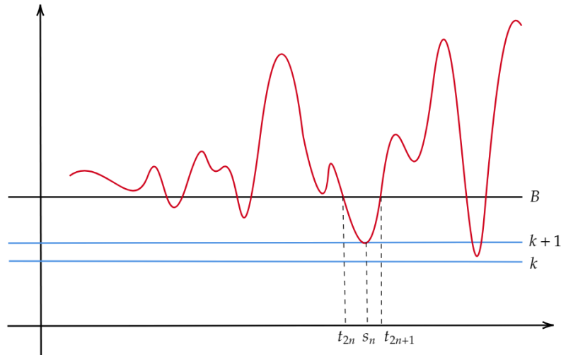
Figura 2.1: Definição das sequências (t_n) e (s_n) .
