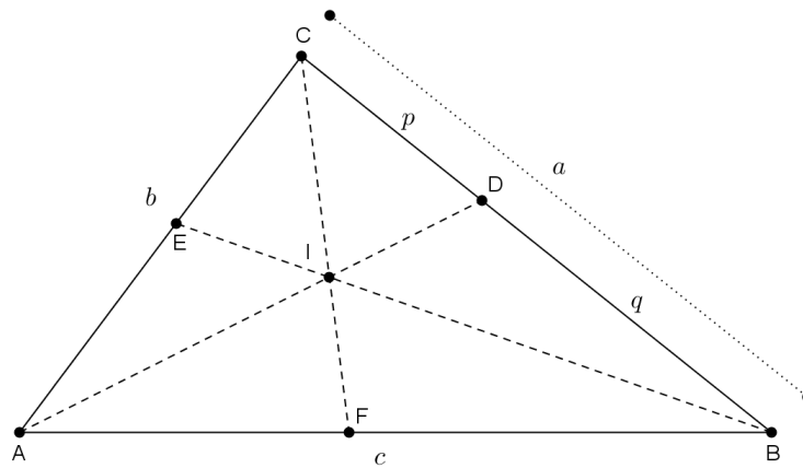
Figura 3.4: Triângulo e seu incentro
