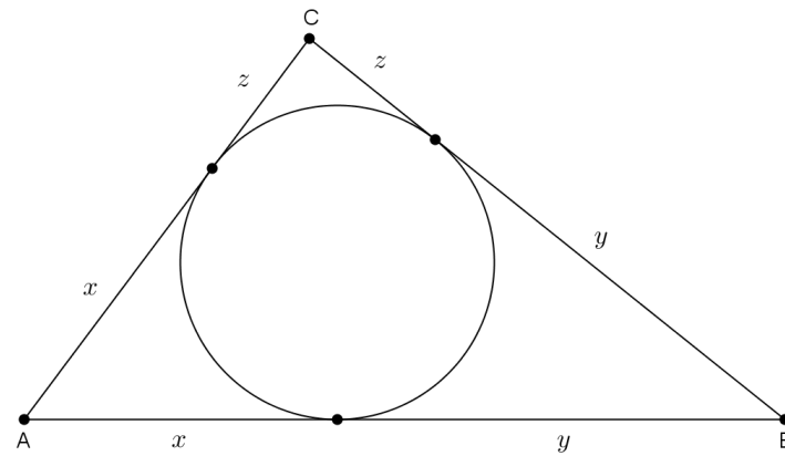
Figura 3.5: Triângulo circunscrito
