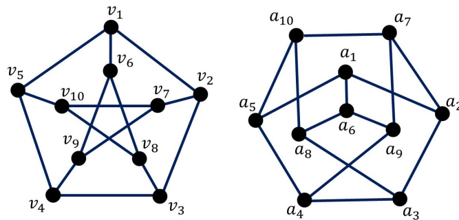
Figura 11 – Grafos Isomorfos
