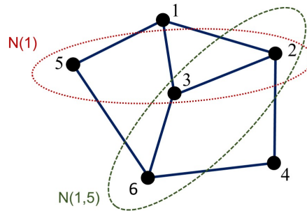
Figura 29 – Vizinhança grafo não orientado
