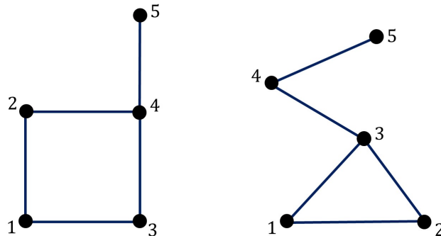
Figura 31 – Grafos para sequência de graus
