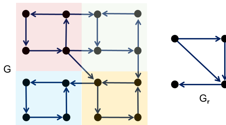
Figura 23 – Grafo reduzido
