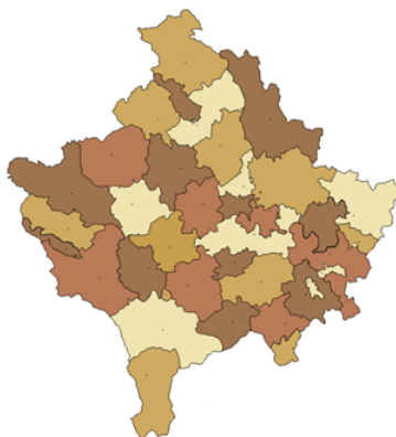
Figura 6 – Mapa colorido com 4 cores
