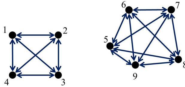
Figura 20 – Grafos desconexos
